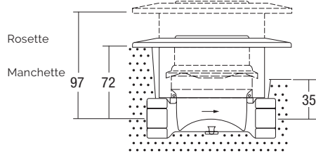
Compensation de la profondeur d'encastrement avec le module de prolongement
