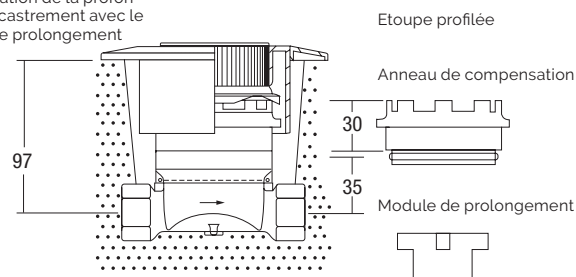
Compensation de la profondeur d'encastrement avec des entretoises
